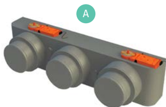
Puszki rozprężne (nawiewna oraz ssąca) + siłownik przepustnicy
